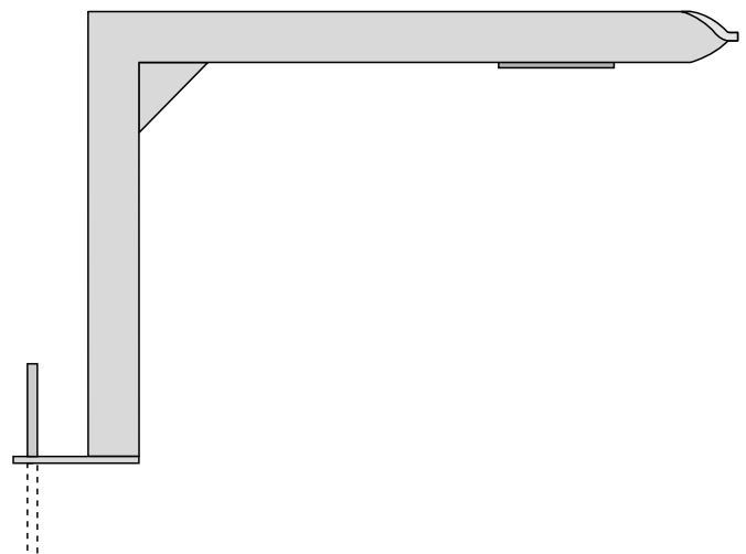
Winkel-Trageanker in der waagrecht Fuge (Seitenansicht)
